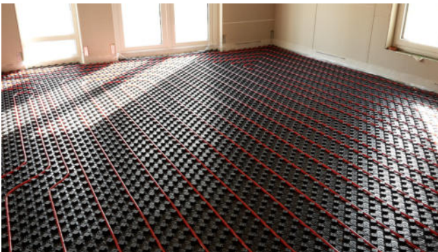
Gruppenraum Fußbodenheizung
