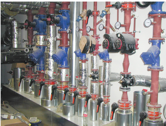
Heizungsverteiler im Kellergeschoss
